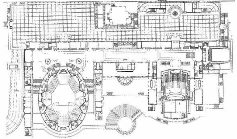
7.00 kotu planı 7.00 level plan
